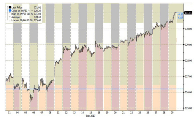
MSCI Europe
